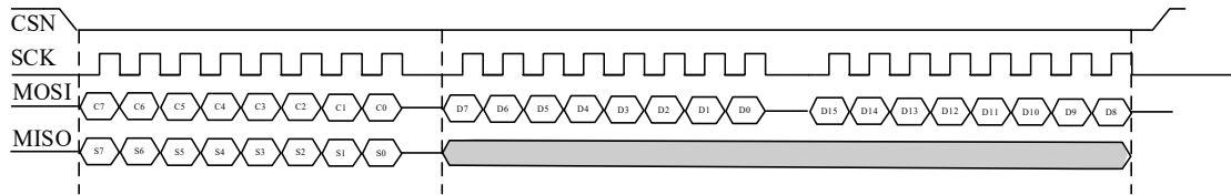
图 5-1 SPI 写操作
