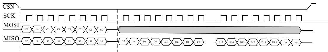
图 5-2 SPI 读操作
