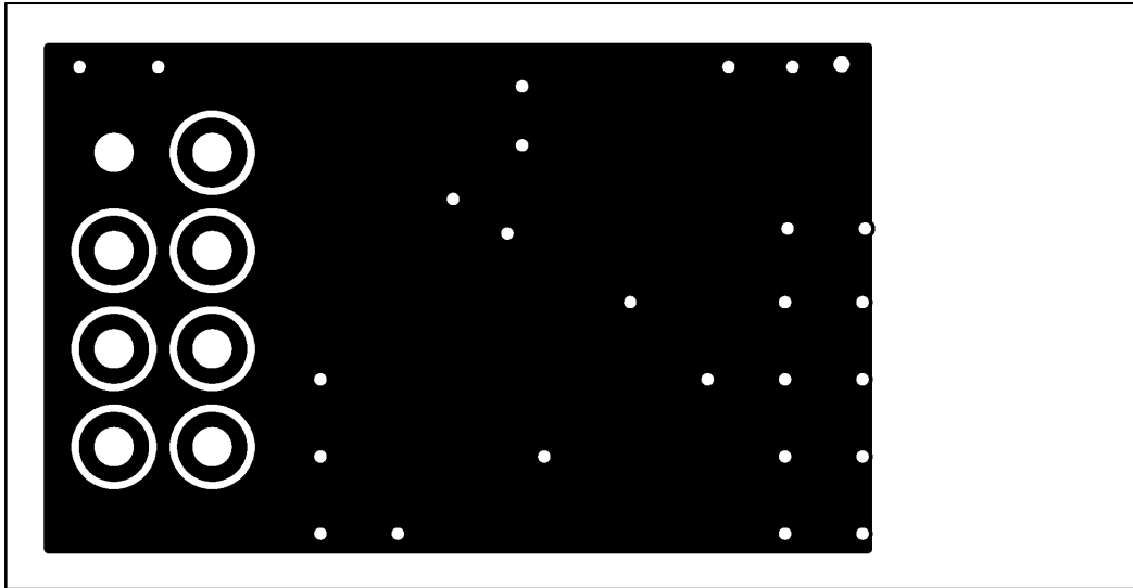
图 9-4 片上天线底层布线图
