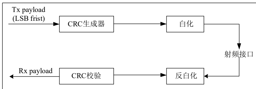
图 4-8 蓝牙数据包数据流
