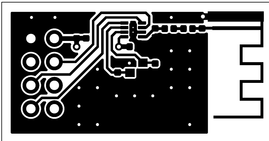
图 9-7 片上天线顶层布线图 (0402 元件)
