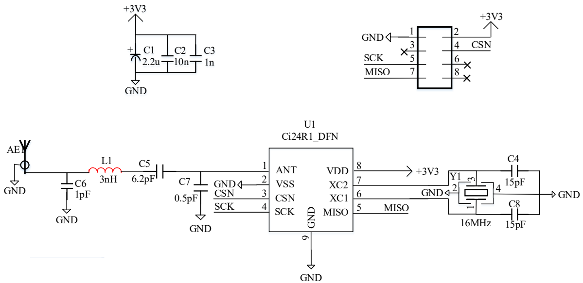
图 9-5 典型应用原理图（DFN-8 封装）
