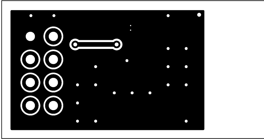
图 9-8 片上天线底层布线图
