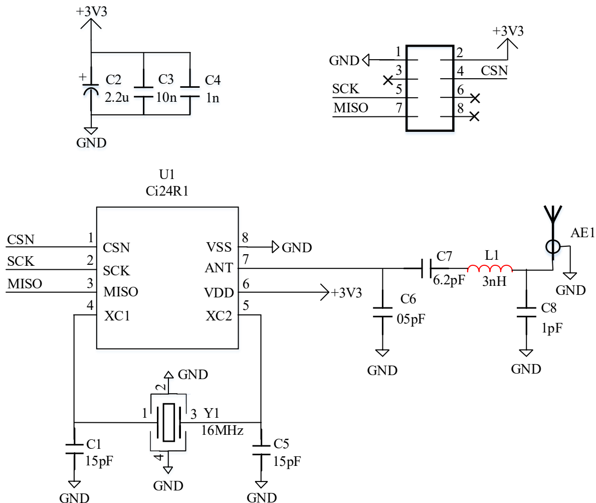
图 9-1 典型应用原理图（SOP-8 封装）
