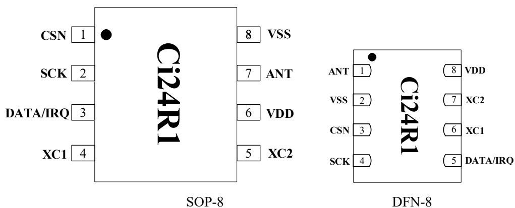
图 2-1 Ci24R1 引脚信息图
