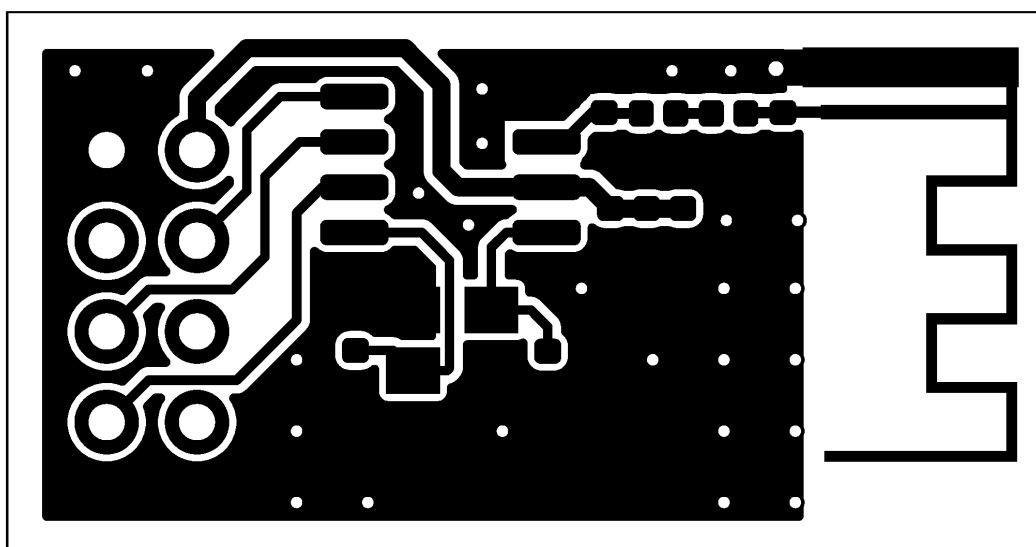
图 9-3 片上天线顶层布线图 (0402 元件)
