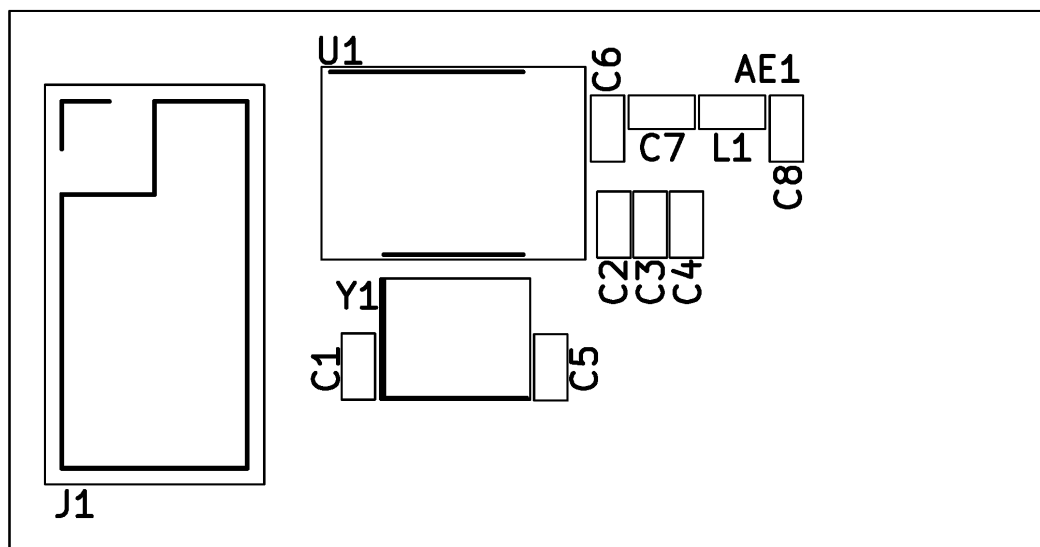
图 9-2 片上天线顶层丝印图 (0402 元件)
