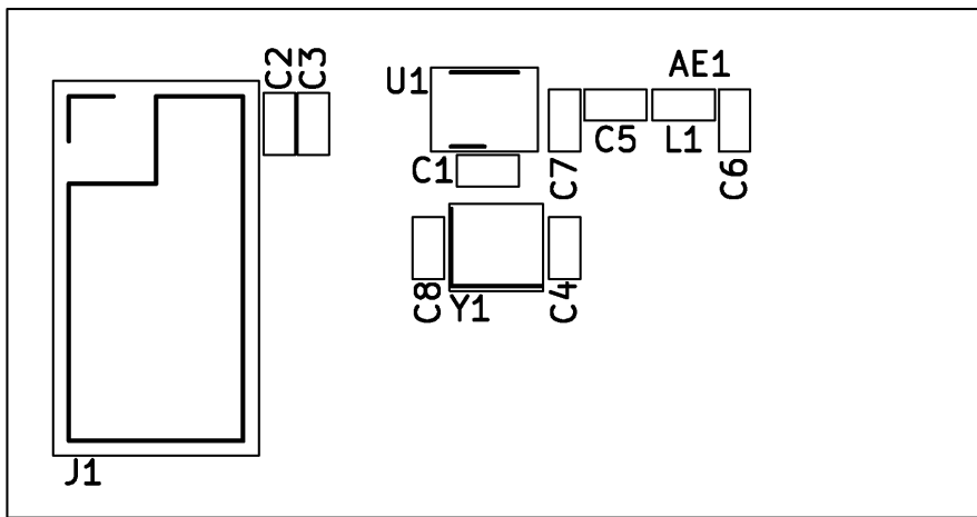
图 9-6 片上天线顶层丝印图 (0402 元件)
